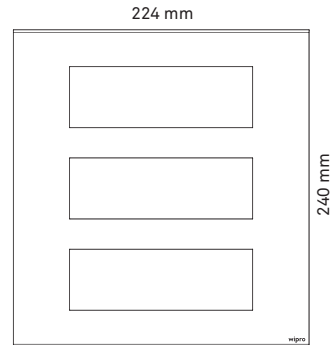
18 Module Plate
